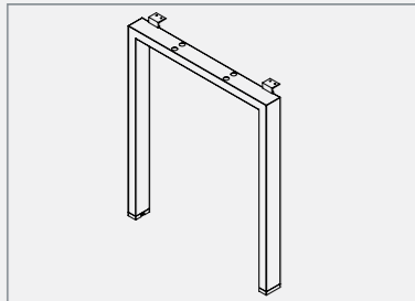
โครงขา U (U Leg) : เหล็กกล่องหน้าตัดขนาด 60x30 มม. หน้า 1.2 มม. ตัดเชื่อมเข้ามุม 45 องศา และทำการพ่นสี Epoxy powder coating
