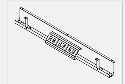
รางร้อยสายไฟและกล่องติดตั้งปลั๊กไฟ (Cable tray & electrical outlet housing) : ช่วยในการจัดการระบบสายไฟต่างๆ ได้อย่างเป็นระเบียบ ผลิตจากเหล็กแผ่นหนา 1 มม. พับขึ้นรูป และกล่องติดตั้งปลั๊กไฟใช้เหล็กแผ่นหนา 1.2 มม. พ่นสี Epoxy powder coating (ไม่รวมอุปกรณ์ไฟฟ้า)
