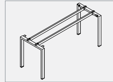
โครงสร้างโต๊ะ (Desk structure) : โต๊ะเป็นระบบคานคู่ ช่วยให้โต๊ะสามารถ รับน้ำหนักได้มากและมีความแข็งแรงสูง โครงสร้างทั้งหมดเป็นโลหะ ทำการพ่นสี Epoxy powder coating
