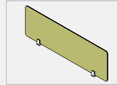
ฉากกั้นหุ้มผ้า (Fabric screen) : ไม้ปาร์ติเกิลบอร์ดหนา 8 มม. เซาะร่องไม้รอบด้าน หรือปาร์ติเกิลบอร์ดหนา 16 มม. หุ้มด้วยผ้า ติดตั้งด้วยตัวจับยึดฉากกั้น
