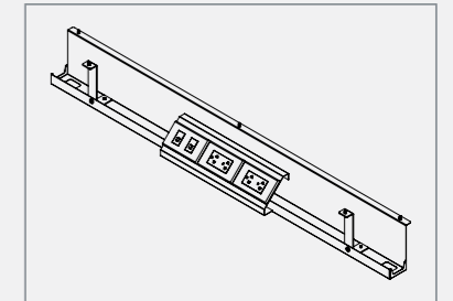
รางร้อยสายไฟและกล่องติดตั้งปลั๊กไฟ (Cable tray & electrical outlet housing) : ช่วยในการจัดการระบบสายไฟต่างๆ ได้ อย่างเป็นระเบียบ ผลิตจากเหล็กแผ่นหนา 1 มม. พับขึ้นรูป และกล่องติดตั้งปลั๊กไฟ ใช้เหล็กแผ่นหนา 1.2 มม. พ่นสี Epoxy powder coating (ไม่รวมอุปกรณ์ไฟฟ้า)
