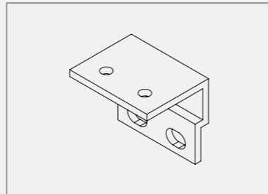
อุปกรณ์ฉากยึดท็อปโต๊ะ (Top support) : อุปกรณ์ฉากยึดจะถูกติดตั้งเข้ากับขาโต๊ะ เพื่อยึดชุดโครงขา เข้ากับแผ่นท็อปโต๊ะเป็น อลูมิเนียมรีดขึ้นรูปพ่นสี Epoxy powder coating
