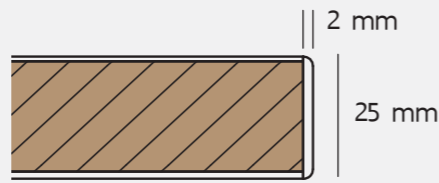
วัสดุ : ปาร์ติเกิลบอร์ดหนา 25 มม. การปิดผิว : ไฮเพรสเซอร์ลามิเนต (HPL) ปิดขอบ : แถบพลาสติกหนา 2 มม.
