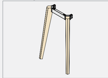
ขา (Leg frame) : เหล็กแผ่นหนา 2 มม. พับขึ้นรูป ตัดเชื่อม ประกอบ และทำการ Water transfer printing ด้วยฟิล์มลายไม้
