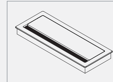
ช่องเสียบปลั๊กไฟจากบนท็อปโต๊ะ (Top access) : ช่วยให้ผู้ใช้สามารถเสียบปลั๊กไฟได้จาก ด้านบนของท็อปโต๊ะได้อย่างสะดวก ด้วยช่อง ขนาด 110 X 290 มม. ผลิตด้วยอลูมิเนียม และเหล็กพ่นสี Epoxy powder coating
