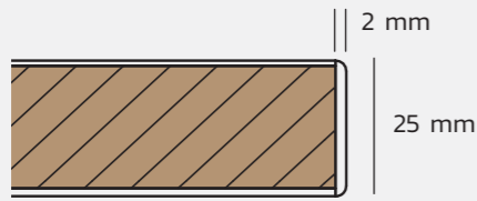
วัสดุ : ปาร์ติเกิลบอร์ด หน้า 25 มม. การปิดผิว : เมลามีน (MFC) ปิดขอบ : แถบพลาสติก หน้า 2 มม.
