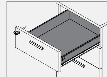
กล่องลิ้นชัก (Drawer box) : กล่องลิ้นชักมี 2 แบบ คือ กล่องลิ้นชักไม้ ผลิตจากไม้ปาร์ติเกิลบอร์ดปิดผิวเมลามีนสีดำ ความหนา 12 มม. และกล่องลิ้นชักเหล็ก ผลิตจากเหล็กแผ่นหนา 0.7 และ 1 มม. พับขึ้นรูป พ่นสี Epoxy powder coating สีดำ ติดตั้งกับรางลิ้นชักแบบรางลูกปืน
