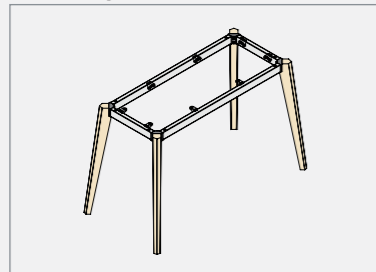
โครงสร้างโต๊ะ (Desk structure) : โต๊ะเป็นระบบคานรอบ ช่วยให้โต๊ะสามารถรับน้ำหนักได้มากและมีความแข็งแรงสูงโครงสร้างทั้งหมดเป็นโลหะ ทำการพ่นสี Epoxy powder coating
