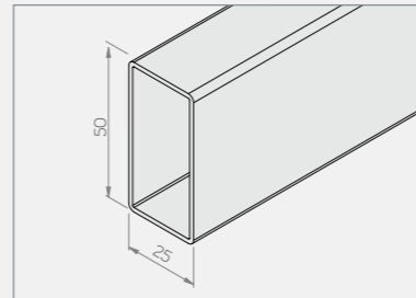
ท่อนคาน (Beam tube) : เหล็กกล่องหน้าตัดขนาด 50x25 มม. หนา 1.2 มม. พ่นสี Epoxy powder coating
