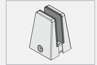
ตัวจับยึดฉากกั้น (Clamp for screen) : ผลิตด้วยกระบวนการฉีดอลูมิเนียมไดแคสติงพ่นสี Epoxy powder coating สามารถใช้ติดตั้งร่วมกับฉากกั้นไม้หุ้มผ้าและกระจกได้
