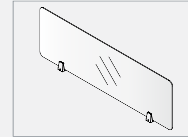
ฉากกั้นกระจก (Glass screen) : -กระจกใสเป็นกระจกธรรมดาเยอรมัน (Float glass) หนา 6 มม. -กระจกฝ้าเป็นกระจกธรรมดาเยอรมัน หนา 6 มม. ทำฝ้าโดยการพ่นทราย (Sandblasting)
