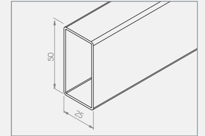
ท่อนคาน (Beam tube) : เหล็กกล่องหน้าตัดขนาด 50x25 มม. หน้า 1.2 มม. พ่นสี Epoxy powder coating
