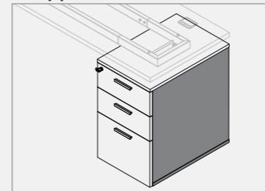
โครงตู้และหน้าบาน (Body & front) : โครงตู้เป็นไม้ปาร์ติเกิลบอร์ดปิดผิว เมลามีนความหนา 16 มม. ท็อปตู้เป็นไม้ ปาร์ติเกิลบอร์ดปิดผิวเมลามีนความหนา 25 มม.
