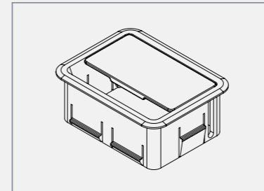
ช่องร้อยสายไฟ (Grommet) : ช่วยในการจัดการร้อยสายไฟบนท็อปโต๊ะ วางร้อยสายไฟได้อย่างเป็นระเบียบ เหมาะกับ การร้อยสายไฟที่ไม่จำเป็นต้องถอดเข้าออก บ่อยๆ ติดตั้งทางซ้ายและขวา ของท็อปโต๊ะ ผลิตด้วยพลาสติก ABS ฉีดขึ้นรูป
