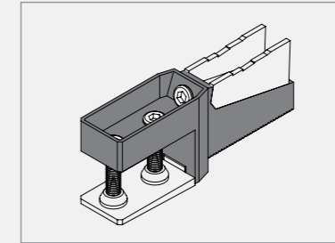
ชุดอุปกรณ์ยึดจับคานเข้ากับโครงขา (Beam clamp) : อุปกรณ์สำหรับจับยึดคานเข้ากับขาโต๊ะ ผลิตด้วยกระบวนการฉีดอลูมิเนียมไดแคสตีง พ่นสี Epoxy powder coating
