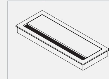
ช่องเสียบปลั๊กไฟจากบนท็อปโต๊ะ (Top access) : ช่วยให้ผู้ใช้สามารถเสียบปลั๊กไฟจากด้านบนของท็อปโต๊ะได้อย่างสะดวก ด้วยช่องขนาด 110 X 290 มม. ผลิตด้วยอลูมิเนียมและเหล็กพ่นสี Epoxy powder coating
