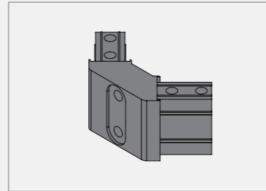
ข้อต่อขา (Corner joint) : ข้อต่อขา ผลิตด้วยกระบวนการฉีดอลูมิเนียมไดแคสติง (Aluminium die-casting) และทำการพ่นสี Epoxy powder coating สีเทา
