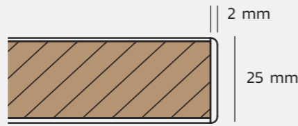
วัสดุ : ปาร์ติเกิลบอร์ด หน้า 25 มม. การปิดผิว : ไฮเพรสเชอร์ลามิเนต (HPL) ปิดขอบ : แถบพลาสติก หน้า 2 มม.
