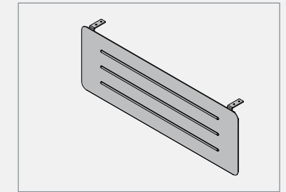
แผ่นบังตาเหล็ก (Steel modesty panel) : แผ่นเหล็กหนา 1.2 มม. พับขึ้นรูป พ่นสี Epoxy powder coating ติดตั้งด้วยชุดอุปกรณ์จับยึดแผ่นบังตา
