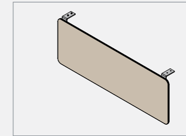
แผ่นบังตาไม้ (Wooden modesty panel) : ปาร์ติเกิลบอร์ดหนา 16 มม. ปิดผิวด้วยเมลามีนหรือไฮเพรสเซอร์ลามิเนต ปิดขอบด้วยแถบพลาสติกหนา 1 มม. รอบด้าน ติดตั้งด้วยชุดอุปกรณ์จับยึดแผ่นบังตา
