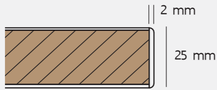
วัสดุ : ปาร์ติเกิลบอร์ดหนา 25 มม. การปิดผิว : เมลามีน (MFC) ปิดขอบ : แถบพลาสติกหนา 2 มม.
