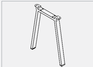
โครงขา H (H Leg) : เหล็กกล่องหน้าตัดขนาด 60x30 มม. หน้า 1.2 มม. ตัดเชื่อม และทำการพ่นสี Epoxy powder coating
