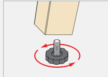
ชุดขาปรับระดับ (Levellor set) : ขนาดเส้นผ่านศูนย์กลาง 24 มม. เป็นพลาสติก ABS ฉีดขึ้นรูป ช่วยในการปรับขาโต๊ะให้มีความสมดุลกัน ในกรณีที่พื้นไม่เรียบหรืออยู่ในระดับเดียวกัน สามารถปรับได้ไม่เกิน 10 มม.
